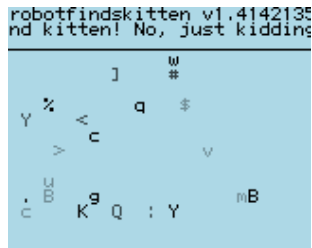
Figure 11.17.: Robotfindskitten
